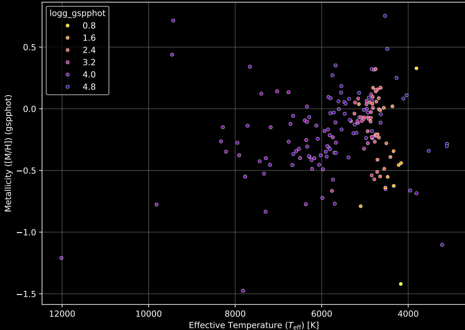
APOGEE DR17 Field: [CVZTILE_092+20_btx] Stellar Population Parameters (n= 175)
